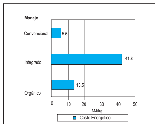
Figura 3. Costo energético unitario de un viñedo Cabernet Sauvignon bajo tres sistemas de manejo.
