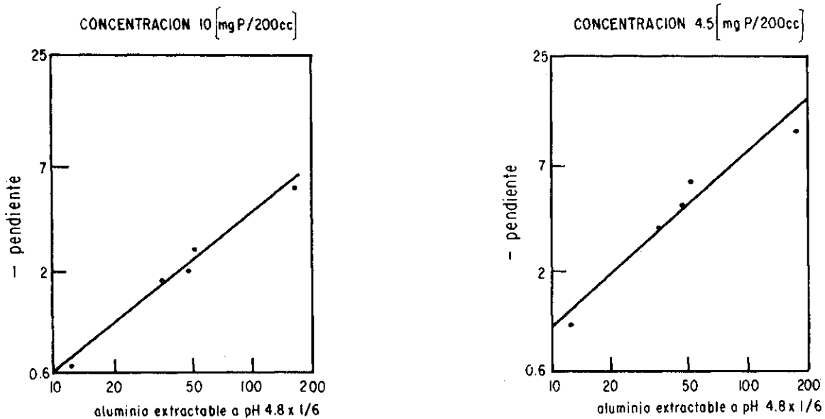
Figura 3.- Influencia del Aluminio extractable a pH 4.8 de los suelos
