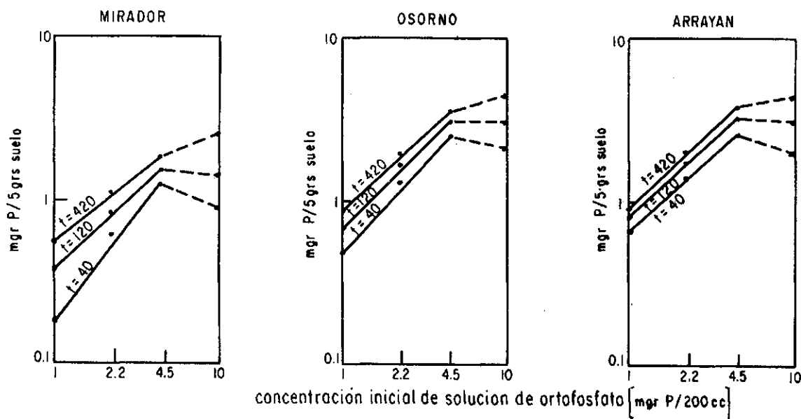
Figura 5.- Isothermas de Adsorción de Freundlich
