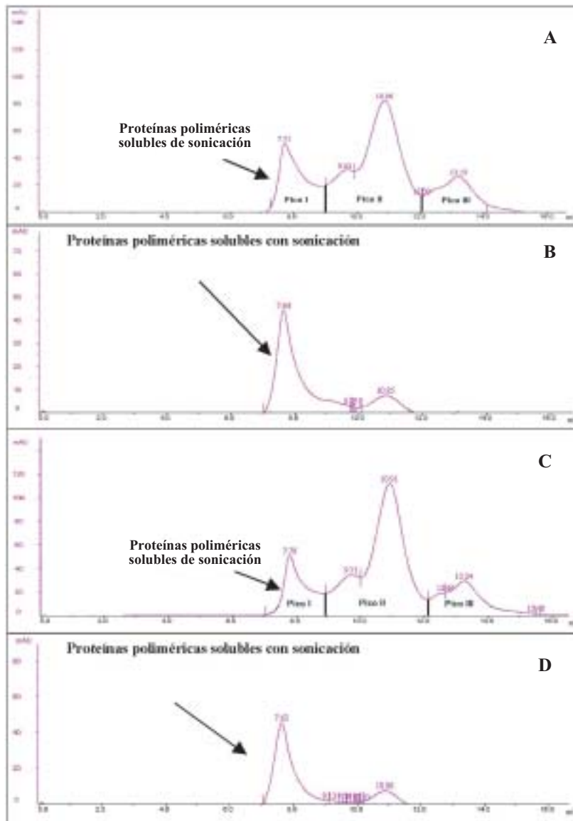
Pico I: proteínas poliméricas, Pico II: gliadinas, Pico III: proteínas no gluten (albúminas y globulinas).
