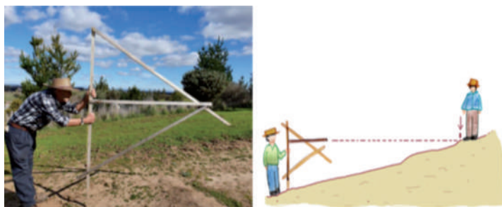
Figura 2. Uso de la mira.
