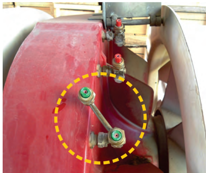
Figura 1. Multiplicador de gota para aumentar el número de boquillas y cubrimiento en un pulverizador hidroneumático.
