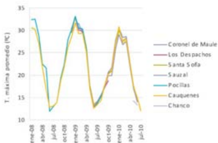
GRAFICO 9. Temperatura máxima promedio registrada en seis estaciones meteorológicas durante tres años.
