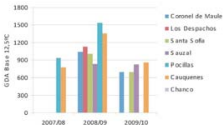
GRAFICO 17: Acumulación de grados día (base 12,5°C) acumulados en Cauquenes durante tres años.
