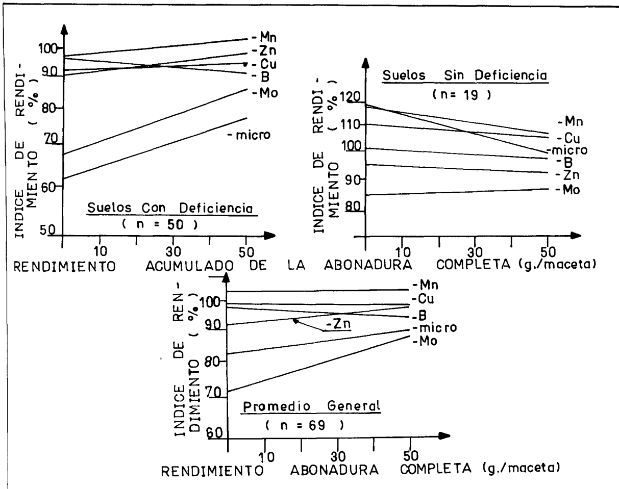
FIGURA 1. Líneas de fertilidad promedio obtenidas para 5 micronutrientes con Trifolium pratense . Arauco FIGURE 1. Average fertility lines, obtained with Trifolium pratense , for five micronutrients. Arauco Province.
