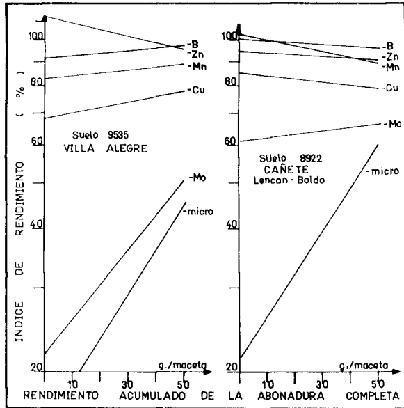
FIGURA 2. Deficiencia múltiple, de varios microelementos, que excluye al B. Arauco. FIGURE 2. Multiple microelements deficiency, that excludes boron. Arauco Province.
