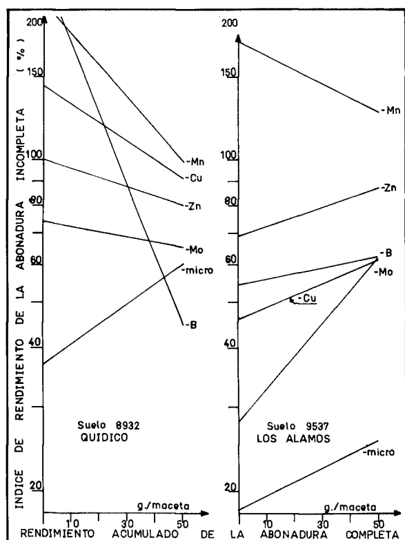
FIGURA 3. Efecto depresivo del Mn (9537) o del Mn, B y Cu (8932) en suelos con deficiencia múltiple. Arauco.
