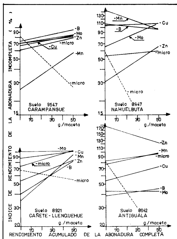
FIGURA 4. Deficiencia múltiple, detectada con trébol rosado (—) y con ballica (---), cuando se omiten varios microelementos. Arauco.
