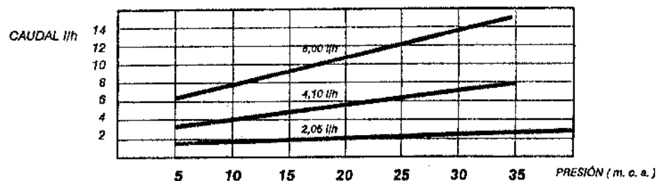
Figura 5. Relación caudal versus presión para goteros de 2,4 y 8 litros por hora.
