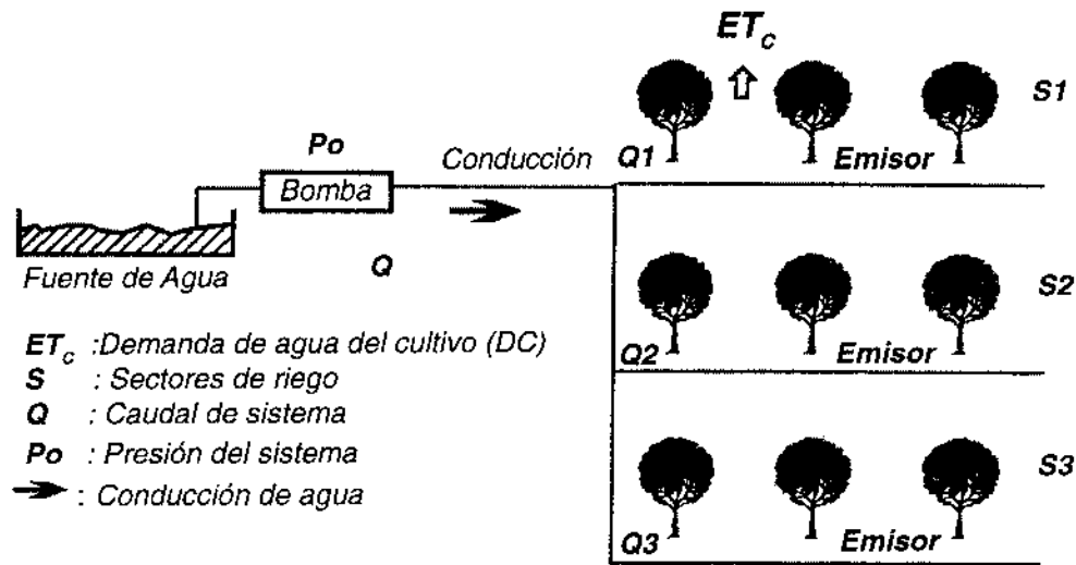
Figura 3: Esquematización de los criterios a considerar en el diseño de un riego presurizado.
