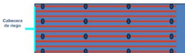
Figura 11.5. Aforo de emisores con probeta graduada y distribución de los puntos de medición.
