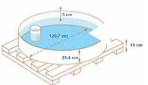
Figura 11.2. Bandeja de evaporación.
