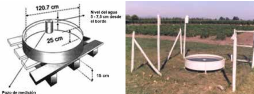
Figura 6.2. Evaporímetro de bandeja Clase A.
